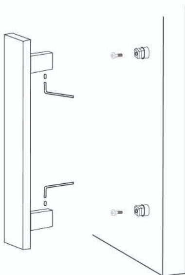
Συναρμολόγηση με βουλόνι Bolt assembly
